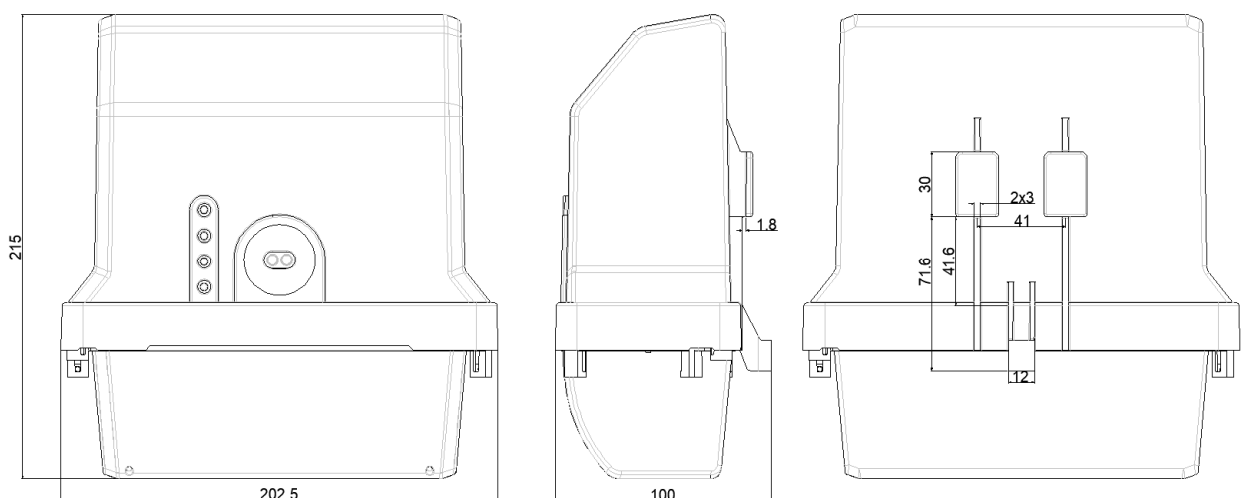
Рисунок 11 – Габаритные и присоединительные размеры счетчика архитектуры «Сплит»
