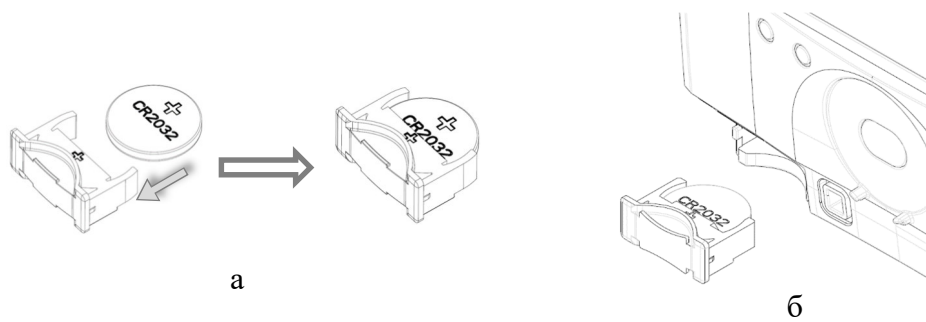
Рисунок 14 – Замена резервного элемента питания счетчика в корпусе типа SP31
