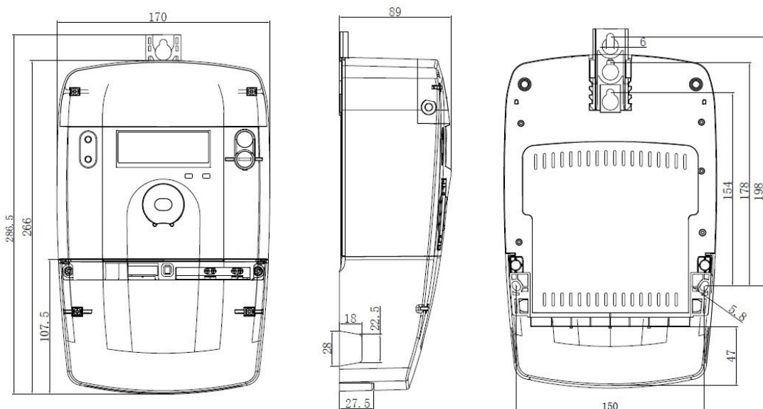
Рисунок 9 – Габаритные и присоединительные размеры счетчика
