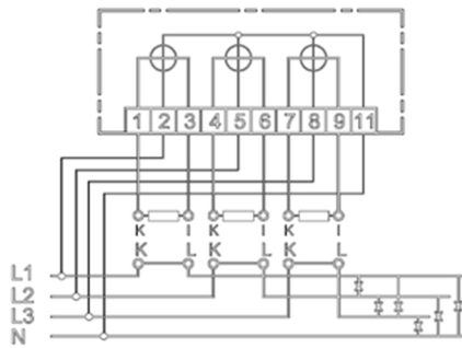
Рисунок 6 – Маркировка схемы включения счетчика трансформаторного типа
