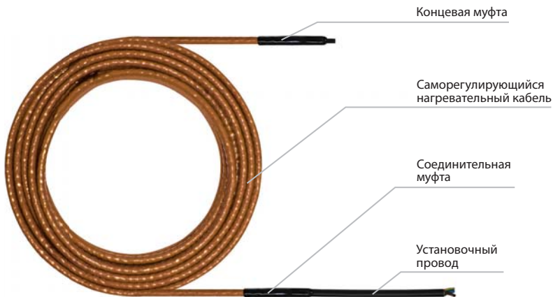
Рис. 1 Конструкция нагревательной секции
